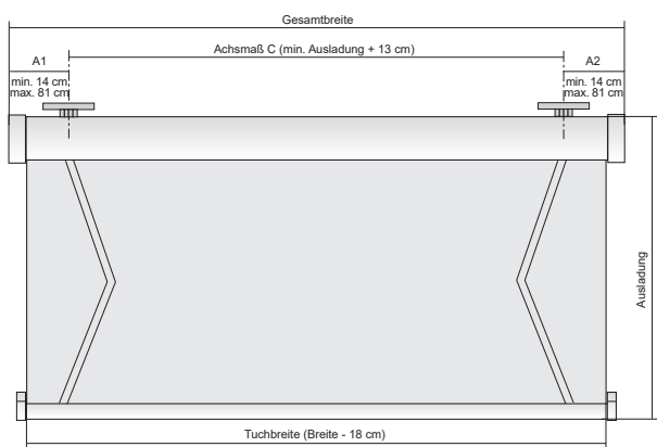
Markise mit 2 Gelenkarmen
