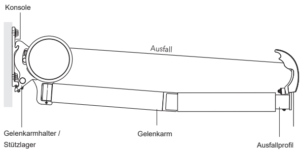
Anzahl Konsolen, Gelenkarme und Stützlager
