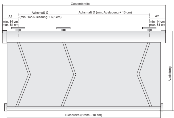
Markise mit 3 Gelenkarmen, in linker oder rechter Ausführung
