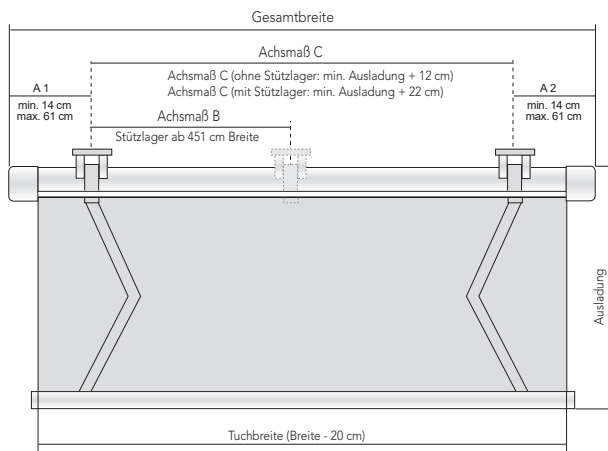
Standard-Achsmaß A1/A2 in cm bei Montage auf Beton
